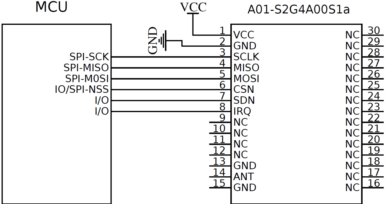
图 5-1 推荐连接图
