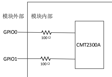
图 5-4 GPIO0、GPIO1 引脚局部连接示意图
