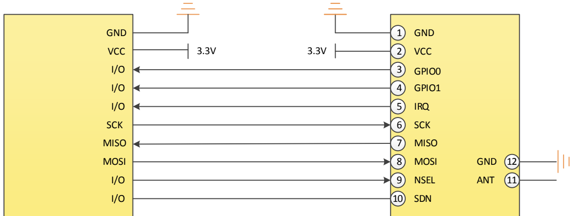
图 5-1 推荐连接图
